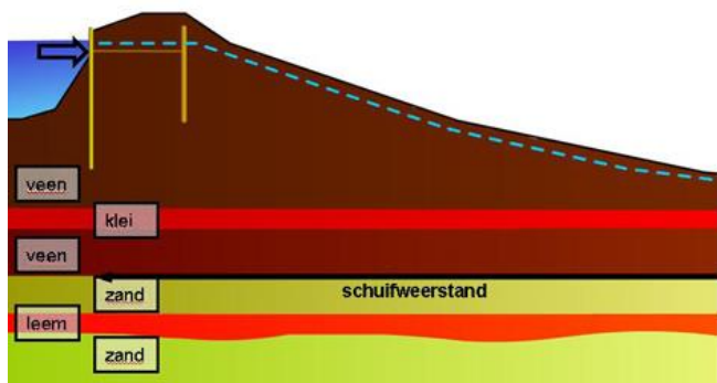
Figuur 3.8: Waterkeringen in de regio Gooi en Vechtstreek. (Bron: Legger Waterkeringen, Waterschap Amstel, Gooi en Vecht)
